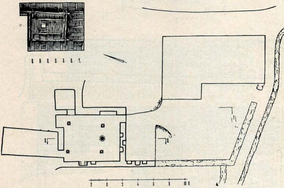
Հացատան կոմպլեքս. կտրվածք, առաստաղ և հատակագիծ. Շինուհայր:
