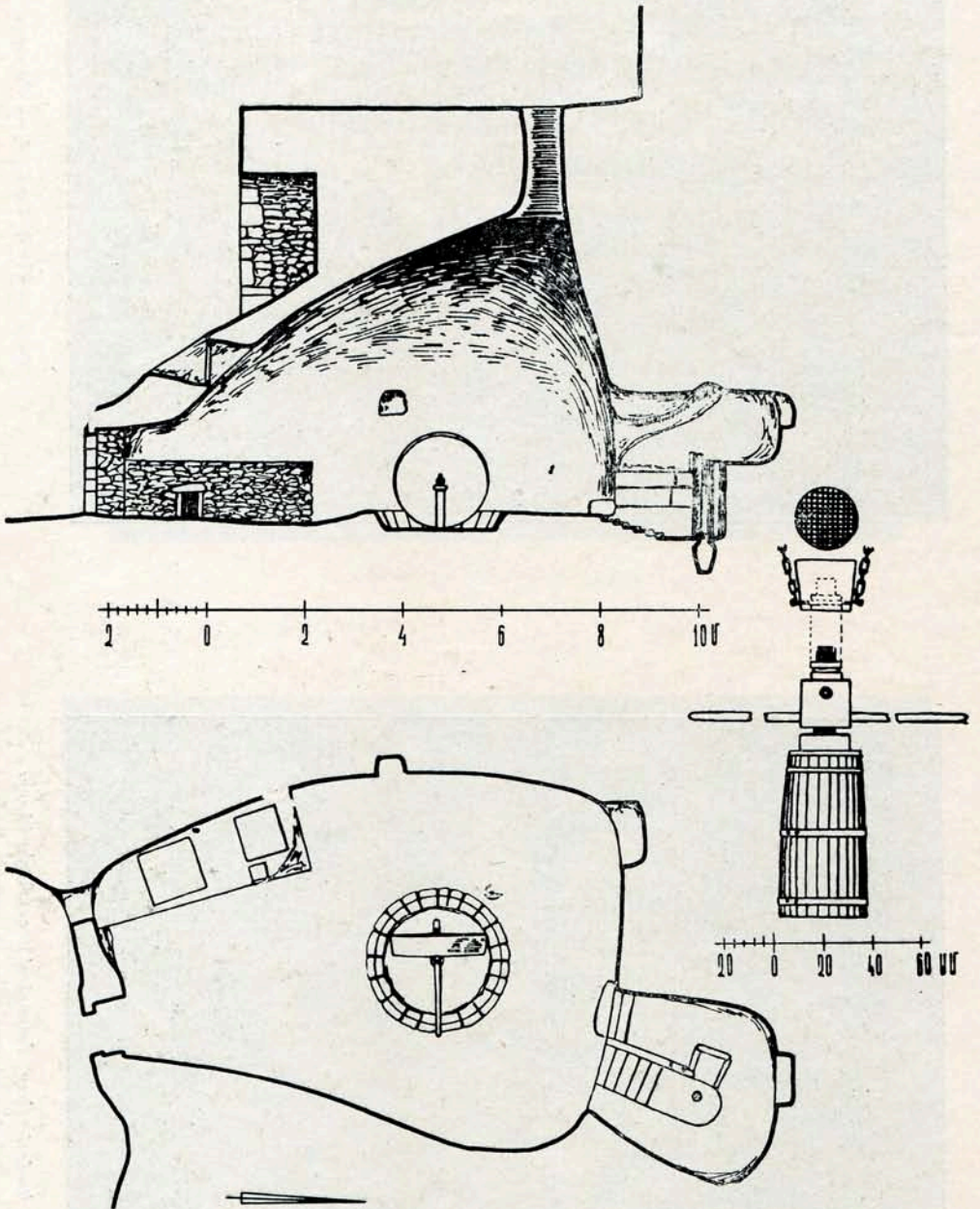
Վիմափոր ձիթահանք. կտրվածք և հատակագիծ. խնձորեսկ:
